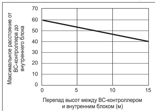
• Зависимость максимального расстояния от ВС-контроллера до внутреннего блока от перепада высот между ними (A)
