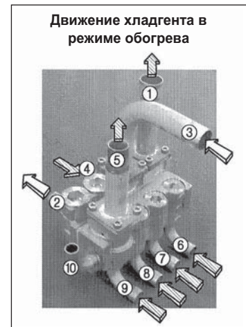
Блок обратных клапанов 1
