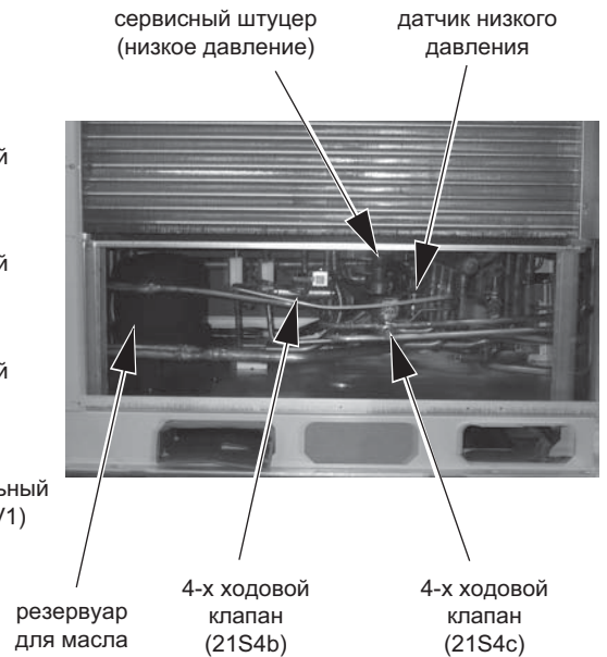
Вид сзади
