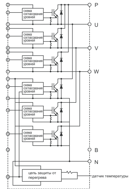
• Структурная схема
