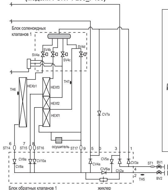
Фрагмент гидравлической схемы (модели PУРУ-P200_P400)
