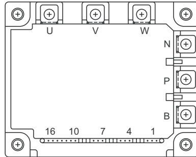
• Внешний вид
