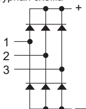
• Структурная схема
