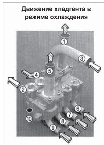
Блок обратных клапанов 1
