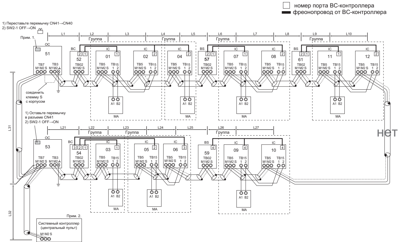
Пример схемы соединений
